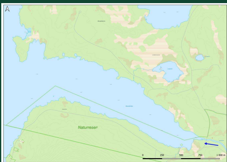
Höljessjöns strandlinje
