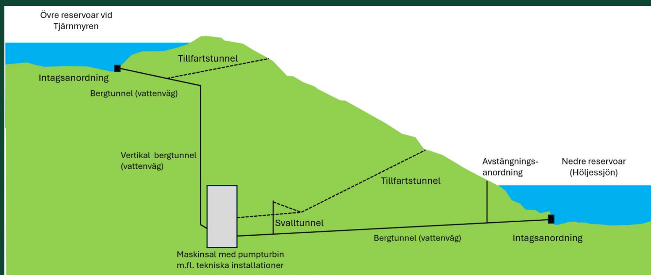
Principiell beskrivning hur ett pumpkraftverk fungerar
